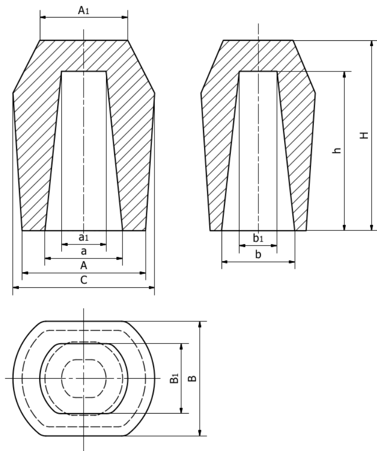
Ilustracja 4: Nasadka owalna OV z podkładką
