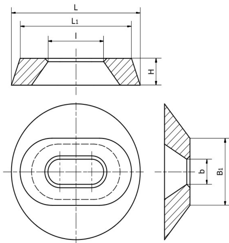
Ilustracja 15: Podkładka O
