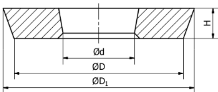
Ilustracja 12: Podkładka C
