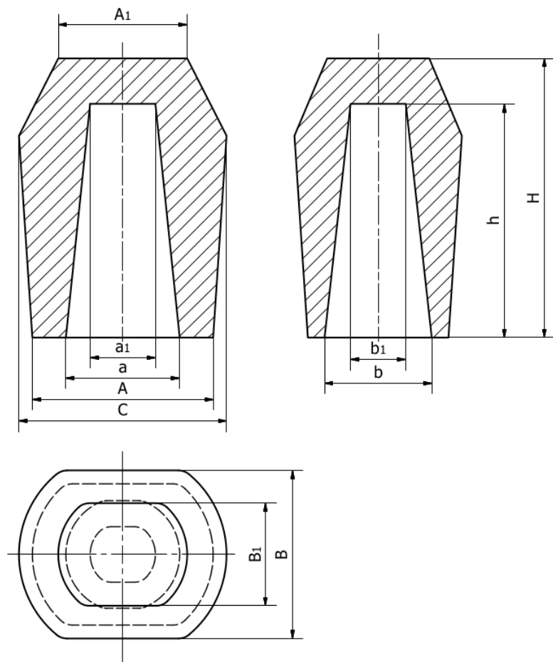
Ilustrace 3: Oválný nástavec OV s podložkou
